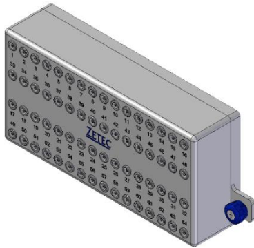
10040441 (ZGN-ACC-DYNARAY-ADPBOX-64LEMO)
